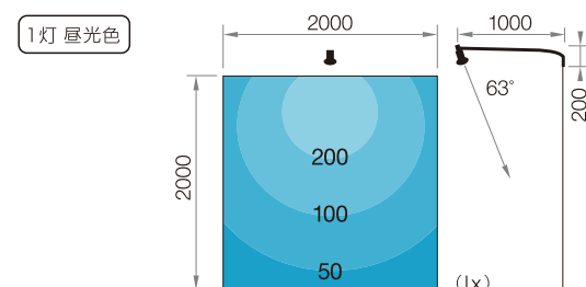
照度分布図
