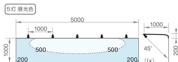
配光曲線図
