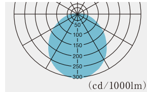
配光曲線図
